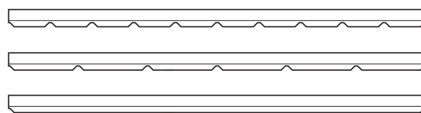
Tværsnit af Troldtekt v-line 2way 6, v-line 2way 10 og v-line 2way blank. Plademål: 25 x 600 x 1200 mm.
