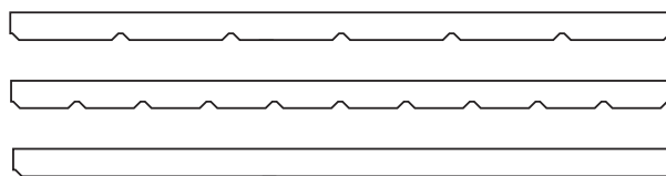
Tværsnit af Troldtekt v-line 1way 6, v-line 1way 10 og v-line 1way blank. Plademål: 25 x 600 x 1200 mm.
