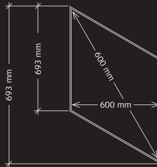
Troldtekt® rhombe hatch
