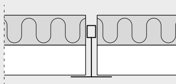
K0- S: Retkantet til synlig T-skinne
